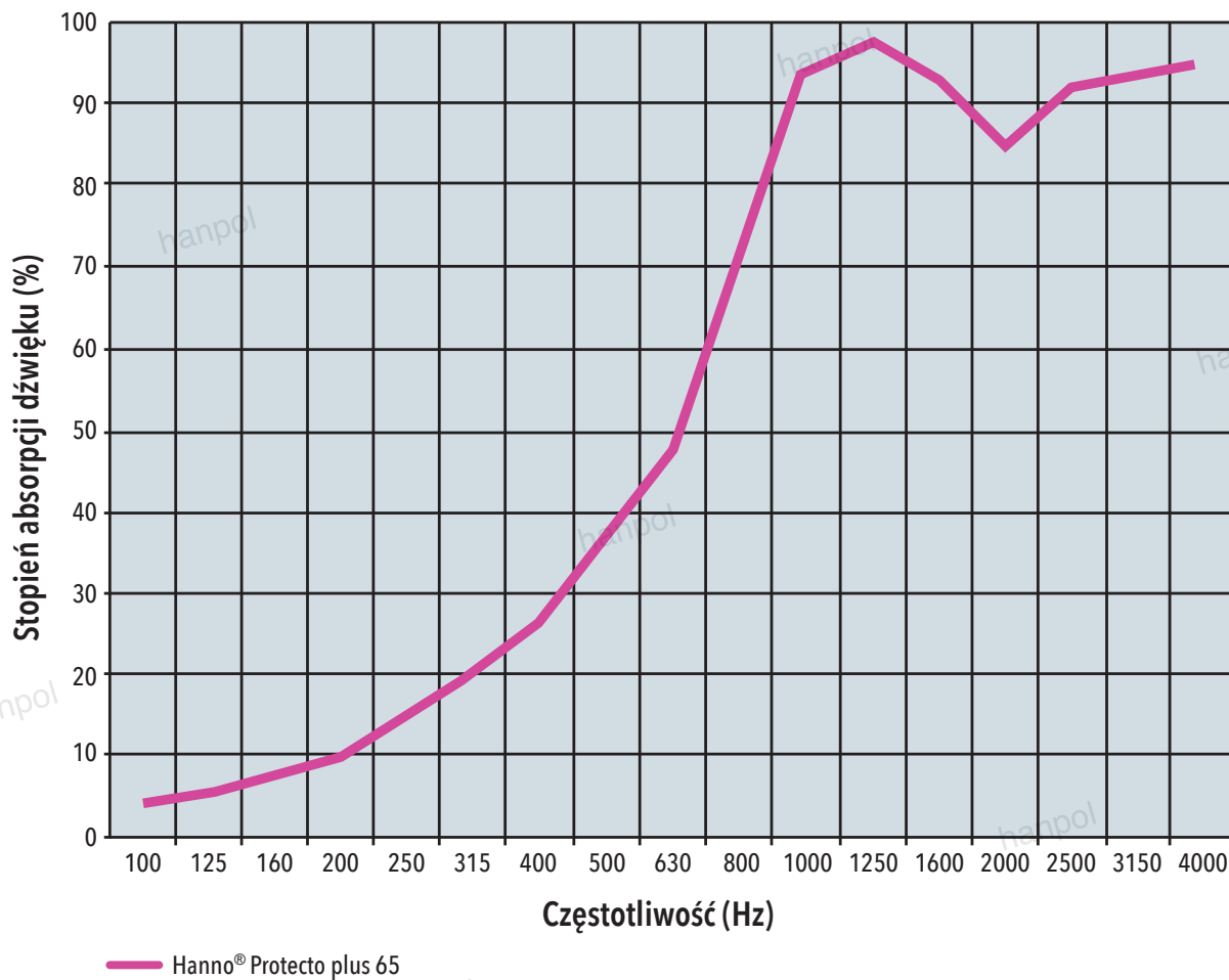
Pomiar współczynnika pochłaniania dźwięków wg DIN-EN-ISO 10534-2
